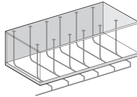
↑ Стандартная самотечная водосточная система здания
